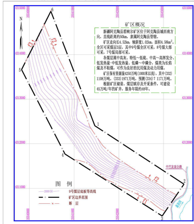
新疆阿克陶县霍峡尔矿区概况说明及示意图
